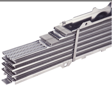
Rohr/ Leitblech Netz aus Kupfer/ Messing Tube and fin core from copper and brass Faisceau traditionnel tubes et ailettes droites en Cu/ Laiton
